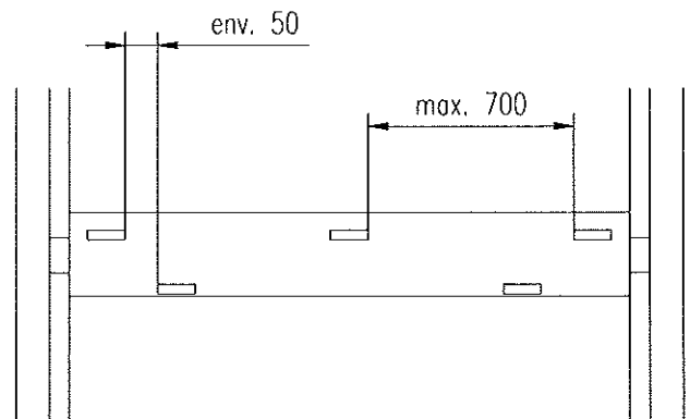
Traverse horizontale d'ouvrant
